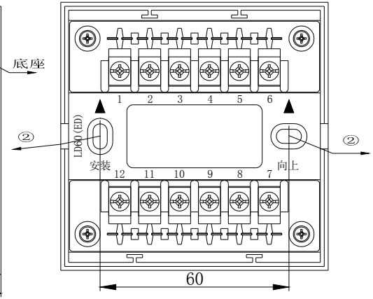
图 3-3 底座图
