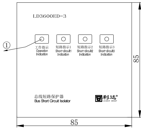
图 3-1 正视图
